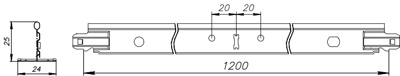
Поперечная направляющая 24/25 L=1200
