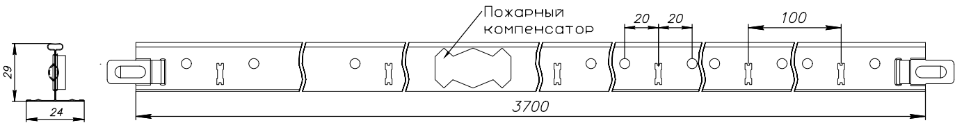
Несущая направляющая 24/29 L=3700
